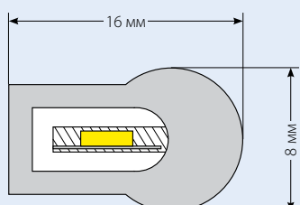
Поперечное сечение светодиодной ленты ULS-N21 NEON
