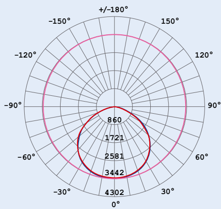
Кривая силы света ассимметричная
